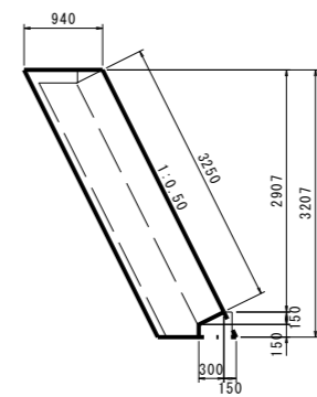
小口止めコンクリート4 S=1:50
