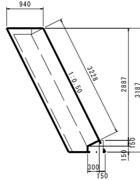
小口止めコンクリート1 S=1:50
