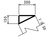
天端コンクリート S=1:20 (裏込めコンクリートなし 1:0.50)
