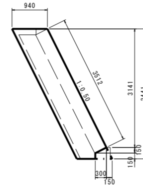
小口止めコンクリート2 S=1:50
