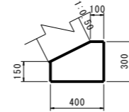
基礎コンクリート S=1:20 (A-1型)
