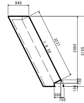
小口止めコンクリート3 S=1:50
