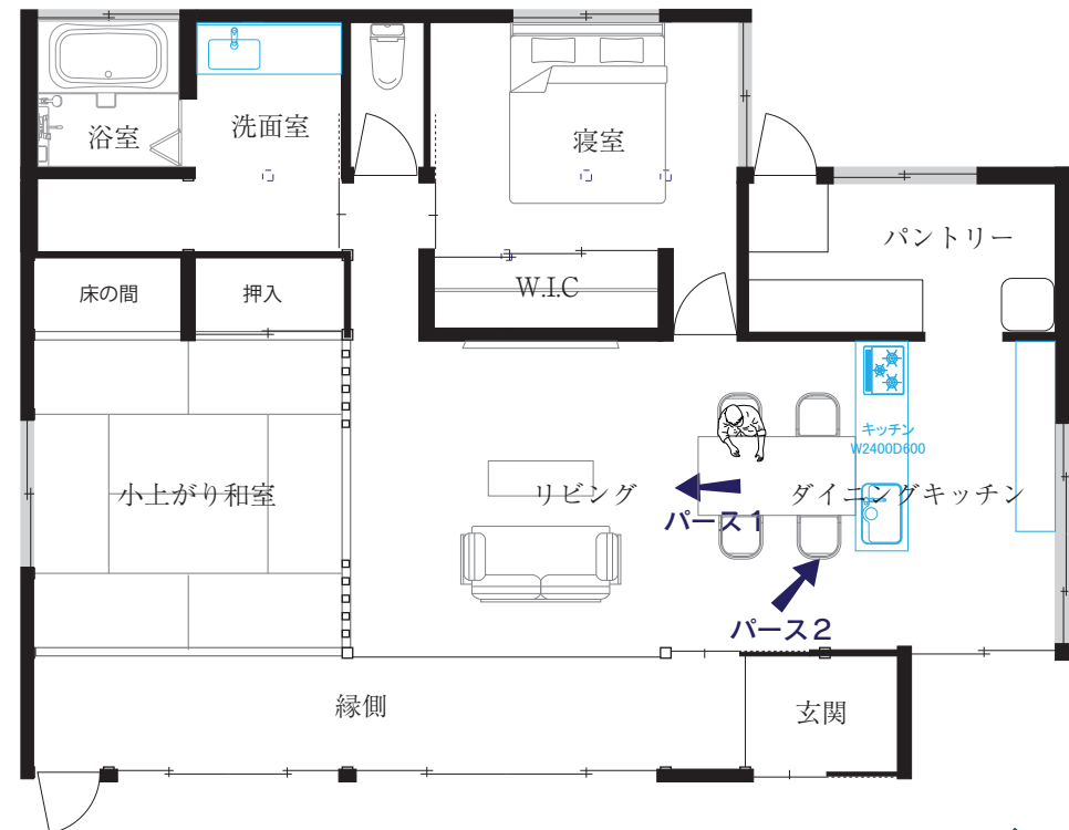
提案平面図
