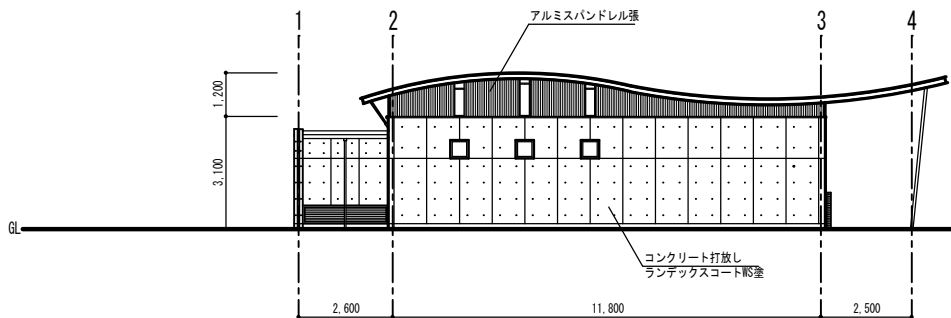
南側立面図 1/100
