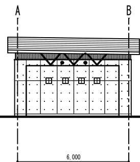
西側立面図 1/100
