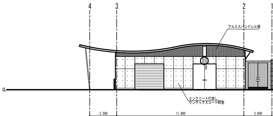
北側立面図 1/100
