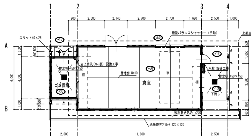
平面図 1/100
