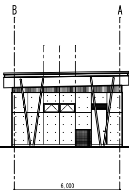
東側立面図 1/100
